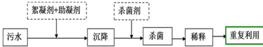
图 4.6-1 污水处理工艺流程
