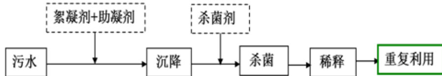
图 4.6-1 污水处理工艺流程
